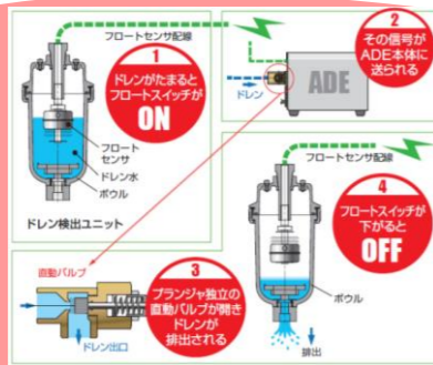
オリオン機械 電磁式オートドレントラップ
