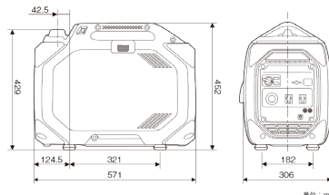
外観寸法図
