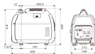
外観寸法図
